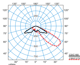
LnPlus 40-AM19L-SLR3/5100-730 6G1 ET (CLO end value)
