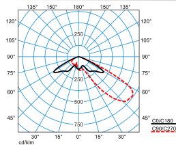
LnPlus 40-AM19L-SLR3/5100-730 6G1 ET (CLO initial value)
