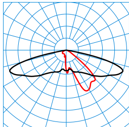
Publisca P1W-AB2L-LRA/2200-730 3G1S ET (CLO end value) TX301712 ■ C0 - C180 ■ C90 - C270 DIN 5040: A30 UTE: 1,00 l DLOR: 100 % ULOR: 0 % CEN Flux Code: 32 69 96 100 100 0 33 67 0
