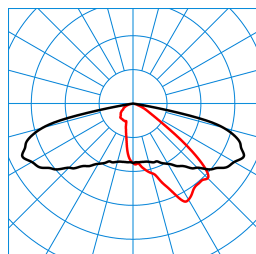
LIQ 50N-AB2L-LR/6800-722 6G1 ET (CLO initial value) TX778045 ■ C0 - C180 ■ C90 - C270 DIN 5040: A30 UTE: 1,00 G DLOR: 100 % ULOR: 0 % CEN Flux Code: 34 71 96 100 100 0 0 0 0
