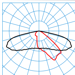
LIQ 50N-AB2L-LR/6800-722 6G1 ET (CLO end value) TX778043 ■ C0 - C180 ■ C90 - C270 DIN 5040: A30 UTE: 1,00 G DLOR: 100 % ULOR: 0 % CEN Flux Code: 34 71 96 100 100 0 0 0 0
