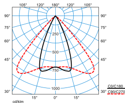
E-Line PRO 78 Grado WRS-DF84 40-827 M40 ET 03 Blank
