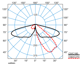
8841LS-UE 360-AB2L/1000-740 2G2 ET (CLO end value)
