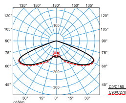
Publisca P1-RB6L-LRA/4200-730 6G1S ET (CLO end value)
