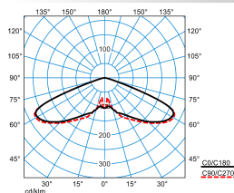
Publisca P1-RB6L-LRA/4200-730 6G1S
