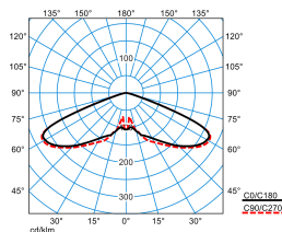
Publisca P1-RB6L-LRA/4200-730 6G1S ET (CLO initial value)
