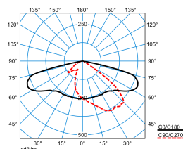
LIQ 70N-AB7L-LR-SLR2/7500-722 8G1 ET (CLO end value)
