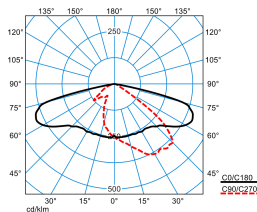
LnPlus 60-AB7L-SLR2/26000-722 24G1 ET (CLO initial value) TX390179
