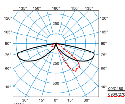
8841 AB2L/700-730 2G2 ETDD (CLO end value)
