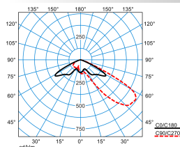
LnPlus 40-AM19L-SLR1/6200-730 6G1 ET (CLO initial value)
