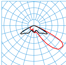
LnPlus 70-AM19L-LR/51000-740 48G1 ET (CLO end value) TX377278
