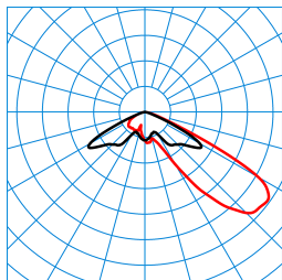
LnPlus 70-AM19L-LR/51000-740 48G1 ET (CLO initial value) TX377398
