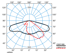
LnPlus60-AB7L24S2-153-7TW-ET-F1 (DWW-CLO end value)
