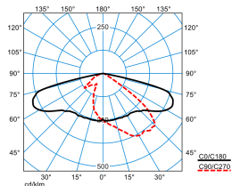
LnPlus60-AB7L24S2-153-7TW-ET-F1 (DSU-CLO end value)
