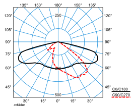
LnPlus60-AB7L24S2-153-7TW-ET-F1 (DSU-CLO initial value)
