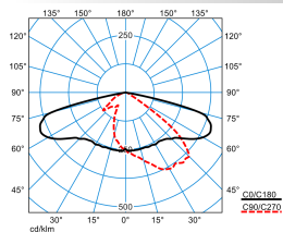
LnPlus60-AB7L24S2-153-7TW-ET-F1 (DWW-CLO initial value)
