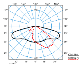
LnPlus60-AB7L24S2-153-7TW-ET-F1 (DCW-CLO end value)
