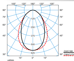
ArimoFit G2 D2 DW19 42-840 ET 01/01
