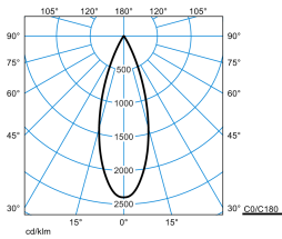
7651 LentyP L-FL 40-EC M39 ETBLE 05 (225)
