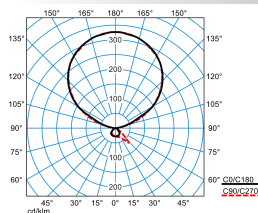
Luceos S G2 PAW-IL 150-830 ETDI 01 +LLWP
