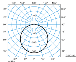
Olisq RWD4 DW 40-830 ETBLE +CAS-S + Olisq RWD4 ZDR 1/2 05
