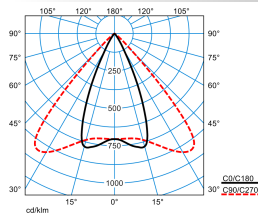
E-Line PRO 78 Grado WRS-DF84 20-EW M50 ET 01 Blank
