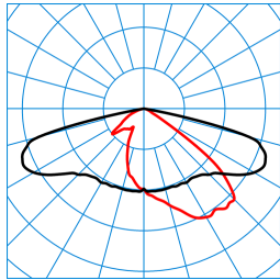
LIQ 70N-AB7L-LRA/12000-730 12G1 ETDD(CLO end value) TX277824
