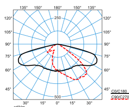
LIQ 70N-AB7L-LRA/12000-730 12G1 ETDD(CLO end value)
