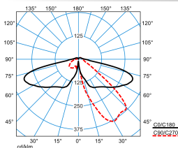
8841LS-UE 260-AB2L/1000-730 2G2 ET (CLO initial value)
