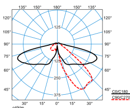
8841LS-UE 260-AB2L/1000-730 2G2 ET (CLO end value)
