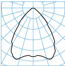
InperiaLP C05 BR25 2700-840 01 + RD-PC TX041602 ■ C0 - C180
