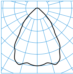
InperiaLP C05 BR25 2700-840 01 + ZN-PC TX041604 ■ C0 - C180
