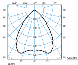
InperiaLP C05 BR25 2700-840 01 + RD-PC TX041602
