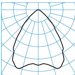
InperiaLP C05 BR25 2700-840 01 + RG-PC TX041603 ■ C0 - C180
