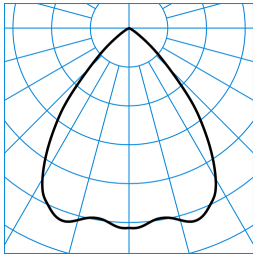
InperiaLP C05 BR25 2700-840 ET 01 TX771661 ■ C0 - C180
