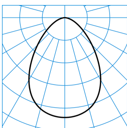
InperiaLP C05 BR25 2700-840 01 + DA-M 01 TX041600 ■ C0 - C180
