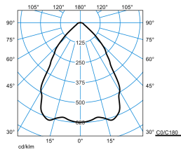
InperiaLP C05 BR25 2700-840 01 + ZN-PC TX041604
