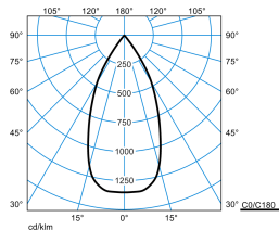
E-Line PRO 78 BV G2 RF-WFL 30-827 M32 ET 03 03
