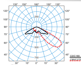
LnPlus 40-AM19L-SLR3/15000-740 12G1 ET (CLO initial value)
