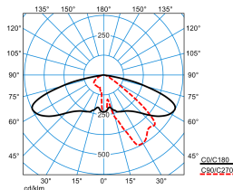
Publisca P1-AB2L-LRA/4200-740 6G1S TX047571 DIN 5040: A30 UTE: 1,00 G DLOR: 100 % ULOR: 0 % CEN Flux Code: 35 74 97 100 100
