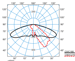
Publisca P1-AB2L-LRA/4200-740 6G1S ET (CLO end value) TX300530 DIN 5040: A30 UTE: 1,00 G DLOR: 100 % ULOR: 0 % CEN Flux Code: 35 74 97 100 100
