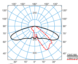
Publisca P1-AB2L-LRA/4200-740 6G1S ET (CLO initial value) TX300631 DIN 5040: A30 UTE: 1,00 G DLOR: 100 % ULOR: 0 % CEN Flux Code: 35 74 97 100 100
