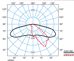
Publisca P3-AB2L-MLLR/16-42-730 4G1 ETDD (CLO end value) TX299960
