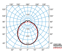
785IP50 DSL35-100 ML 830 L150 10 50
