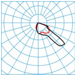
Jovie 70-FR1L-8-68-730-CLO-E
