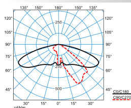
Publisca P2-AB2L/4200-730 6G1S
