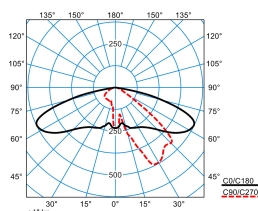
Publisca P2-AB2L/4200-730 6G1S ETDD (CLO end value)
