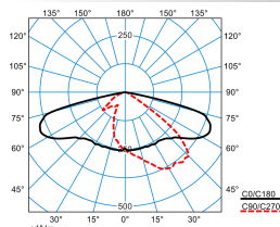
LnPlus 60-AB7L-LR/24000-730 18G1 ET (CLO initial value)
