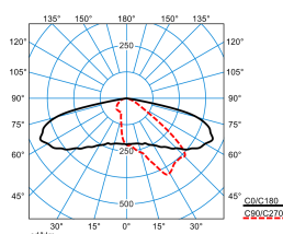
LIQ 50N-AB2L-SLR2/6800-730 6G1 ET (CLO end value)
