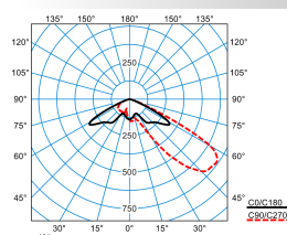
LnPlus 70-AM19L-SLR2/62000-740 48G1 ET (CLO initial value)
