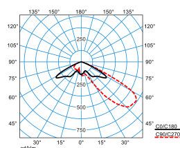
LnPlus 70-AM19L-SLR2/62000-740 48G1 ET (CLO end value)
