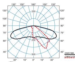
Publisca P3-AB2L/6800-740 6G1 ETDD (CLO end value)
