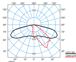
Publisca P3-AB2L/6800-740 6G1
