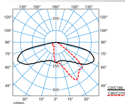
Publisca P3-AB2L/6800-740 6G1 ETDD (CLO initial value)
