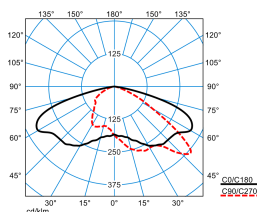
LnPlus 40-AB7L-LR/6200-722 6G1 ET (CLO end value)
