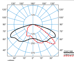
LnPlus 40-AB7L-LR/6200-722 6G1 ET (CLO initial value)
