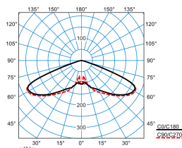
Publisca P1-RB6L-LR/5600-740 6G1S ET (CLO end value)
