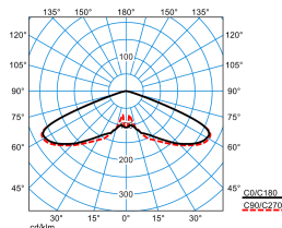
Publisca P1-RB6L-LR/5600-740 6G1S ET (CLO initial value)
