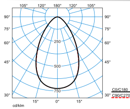
7651IP MironaF TB 130-840ET L150 01ESG (LEO1)
