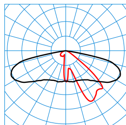
Publisca P2-AB2L/1000-730 2G1S ETDD (CLO end value) TX301689 ■ C0 - C180 ■ C90 - C270 DIN 5040: A30 UTE: 1,00 G DLOR: 100 % ULOR: 0 % CEN Flux Code: 34 70 96 100 100
