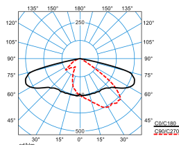
LIQ 70N-AB7L-LR/12000-722 12G1 ET (CLO end value)
