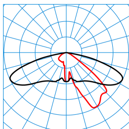
Publisca P1-AB2L-LR/5100-740 6G1S ET (CLO initial value) TX300647 ■ C0 - C180 ■ C90 - C270 DIN 5040: A30 UTE: 1,00 G DLOR: 100 % ULOR: 0 % CEN Flux Code: 35 74 97 100 100
