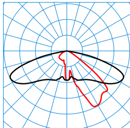
Publisca P1-AB2L-LR/5100-740 6G1S TX047538 ■ C0 - C180 ■ C90 - C270 DIN 5040: A30 UTE: 1,00 G DLOR: 100 % ULOR: 0 % CEN Flux Code: 35 74 97 100 100
