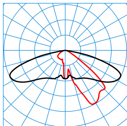
Publisca P1-AB2L-LR/5100-740 6G1S ET (CLO end value) TX301449 ■ C0 - C180 ■ C90 - C270 DIN 5040: A30 UTE: 1,00 G DLOR: 100 % ULOR: 0 % CEN Flux Code: 35 74 97 100 100
