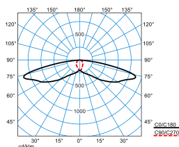
LIQ 50N-SB3L-LR/1800-730 2G1 ET (CLO end value)
