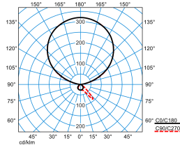
Luceos S-U G3 PAW-IL 300-840 ETDS 03 (LEO1)
