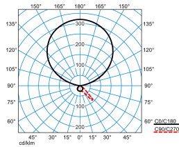
Luceos S-U G3 PAW-IL 300-840 ETDS 03 (LEO2)
