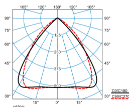
ELINE LN40-110 ML 865 L150 4 20
