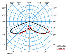
Publisca P1-RB6L-LRA/2400-740 3G1S ET (CLO end value) TX300727 DIN 5040: A20 UTE: 1,00 J DLOR: 100 % ULOR: 0 % CEN Flux Code: 20 57 98 100 100
