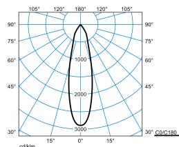
E-Line PRO 78 BV G2 RF-MF 30-EC M39 ET 05 Blank
