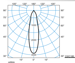
E-Line PRO 78 BV G2 RF-MF 30-EC M39 ET 05 05
