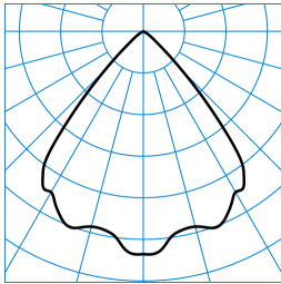
InperiaLP C05 HR25 2700-830 ET 03 TX771355
