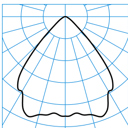
InperiaLP C05 HR25 2700-830 03 + DA 01 TX041774
