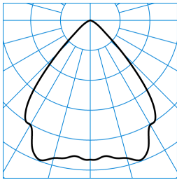
InperiaLP C05 HR25 2700-830 03 + RD-PC ■ C0 - C180 TX041778
