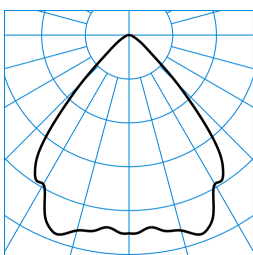
InperiaLP C05 HR25 2700-830 03 + DA 03 TX041775
