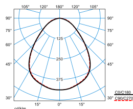
E-Line PRO 78IP50 MironaF B 130-840 ETDD L150 01 Blank (LEO1)
