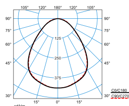
E-Line PRO 78IP50 MironaF B 130-840 ETDD L150 01 Blank IP50 (LEO2)
