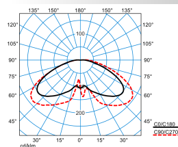
Publisca P1W-RBT-LRA/2200-730 3G1S ET (CLO initial value)
