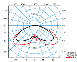
Publisca P1W-RBT-LRA/2200-730 3G1S
