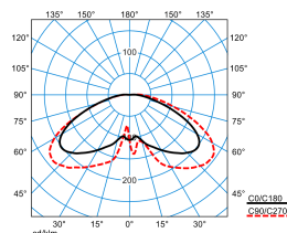
Publisca P1W-RBT-LRA/2200-730 3G1S ET (CLO end value)
