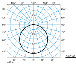
Olisq RWD2 DW 20-840 ET HFS PC + Olisq RWD2 ZDR 1/2 01
