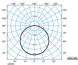
Olisq RWD2 DW 20-840 ET HFS PC + Olisq RWD2 C 01
