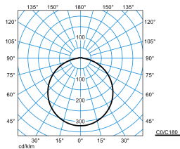
Olisq RWD4 DW 60-840 ET IP54 PC + Olisq RWD4 C 01
