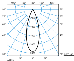
E-Line PRO 78 LentyP L-FL 40-835 M34 ETBLE 03 Blank
