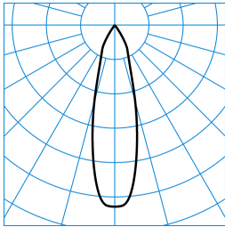
Can G2 3P RF-MF 30-830 M33 ET 01 TX870786
