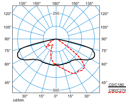
LIQ 70N-AB7L-SLR1/16500-740 12G1 ET (CLO end value) TX777988
